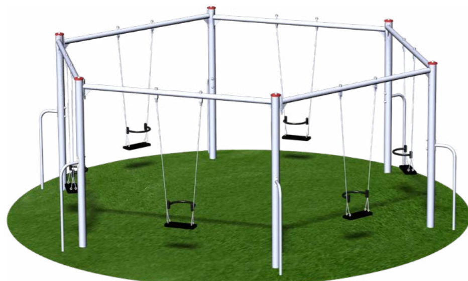
phex6 - 3/10 ans - 6 enfants - 77m 2 - 12850x12300 mm
